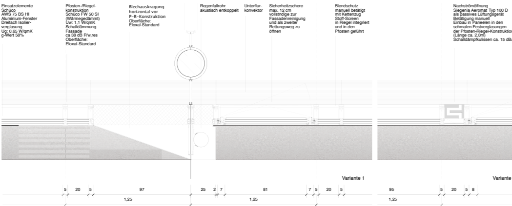
1:10 Schnitt-Detail
